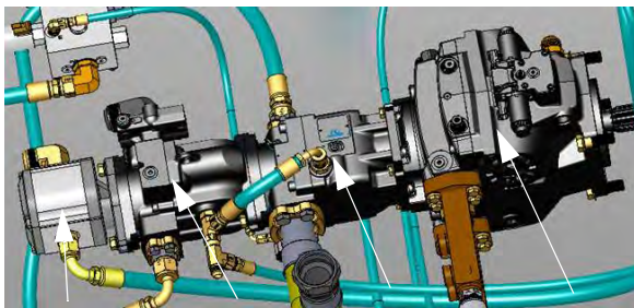
• 齿轮泵 • PC 泵 • LS 泵 • 驱动泵
