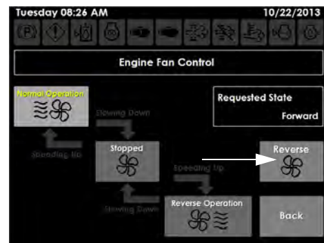
“发动机风扇控制”屏幕
