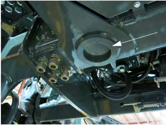
起重吊点保护环 (位于靠近每个立腿的框架上) -典型视图
