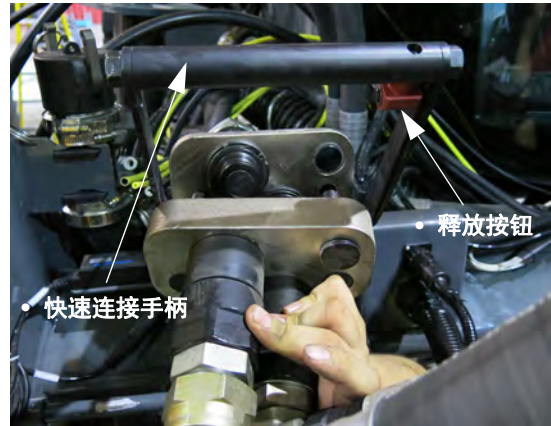
液压多功能联结器总成 (图示机器右侧) - 典型视图
