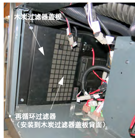
木炭过滤器盖板 （位于驾驶室右侧的室外检修面板背面） - 典型视图
