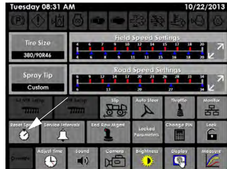
复位喷药按钮 (位于设置页面上)
