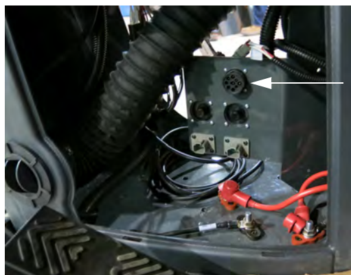
发动机诊断接口 (位于侧控制台的内侧 - 取下前面板后可以够着) - 典型视图
