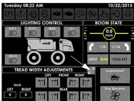
胎面页面按钮 (位于辅助控制器页面上)
