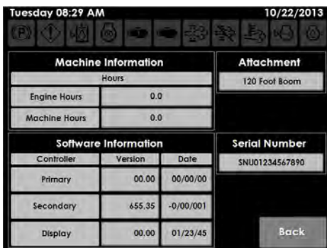
“机器信息”屏幕
