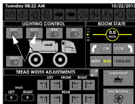
现场照明灯按钮 (位于辅助控制器页面上)
