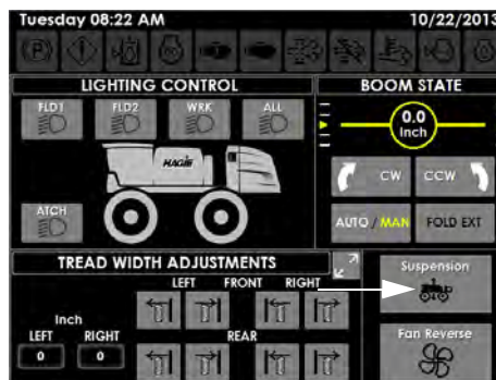
悬架按钮 (位于机器显示屏辅助控制器页面上)
