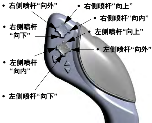
左/右喷杆开关方向 - 典型视图
