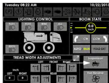
悬架按钮 (位于辅助控制页面)
