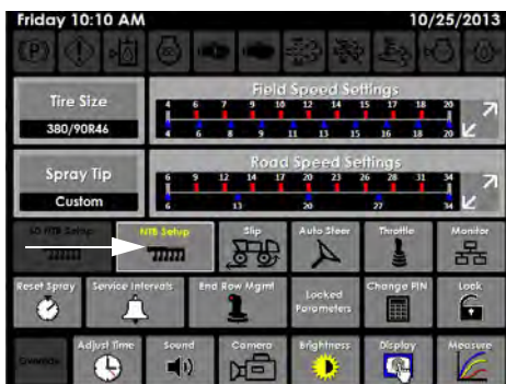
NTB 设置按钮 (位于设置页面上) - 典型视图
