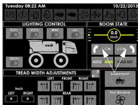
转动命令按钮 (CW/CCW) (位于辅助控制器页面的右侧)
