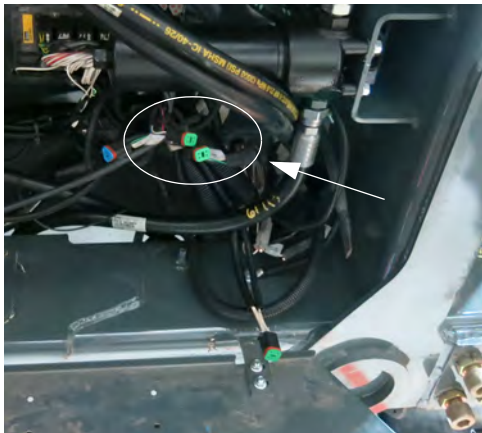
视频摄像头输入接口 （位于驾驶室下方 - 拆除前面板 后可以够着） - 典型视图
