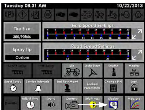
显示按钮 (位于设置页面上)
