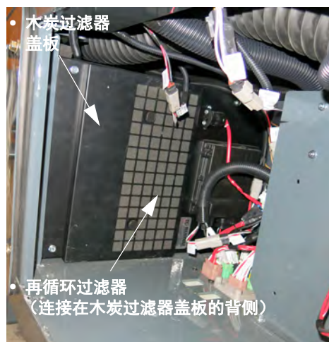
木炭过滤器盖板 (位于驾驶室右侧的室外 检修面板的后侧) - 典型视图
