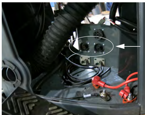
海吉诊断端口 (2) (位于侧控制台的内侧 - 取下前面板后可以够着) - 典型视图
