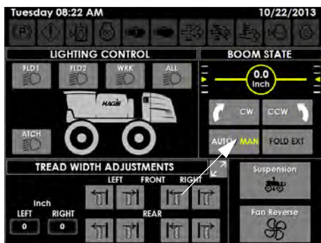
喷杆状态按钮 – 自动/手动 (位于机器显示屏辅助控制器页面)
