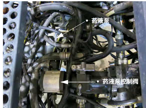
药液泵和药液泵控制阀 - 典型视图 *机器上方的俯视图
