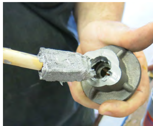
涂防卡润滑剂 - 典型视图
