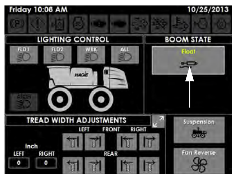
漂浮按钮 (位于辅助控制器页面上)
