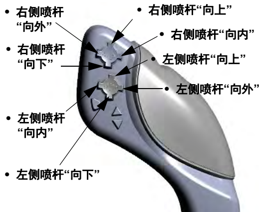
左侧和右侧喷杆开关朝向 - 典型视图
