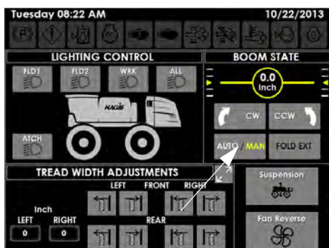
喷杆状态按钮 - 自动/手动 (位于机器显示屏辅助控制器页面上)
