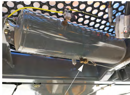
箱放气阀 （位于机器左手侧通道之下） 向下拉来打开 - 典型视图
