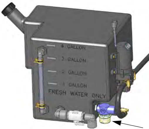
洗手水滤网 (位于靠近洗手水箱底部) - 典型视图
