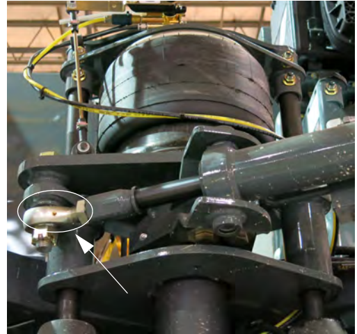
连杆球润润滑脂加油嘴 (位于前立腿上) - 典型视图
