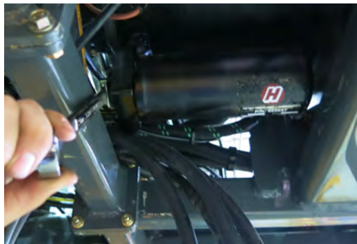
加液泵过滤器 (位于驱动泵之下) - 典型视图
