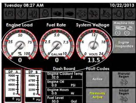
系统量表 (位于机器诊断页面上)
