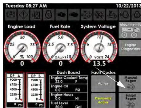
手动再生按钮 (位于机器诊断页面的底部)
