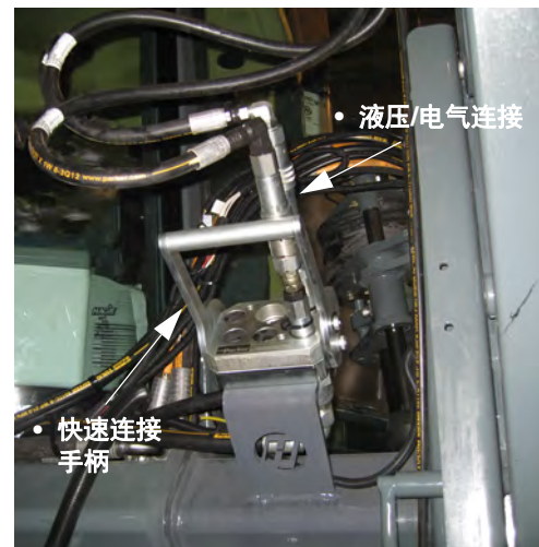
液压/电力多功能联结器总成 - “如已配置” (位于机器左前侧)
