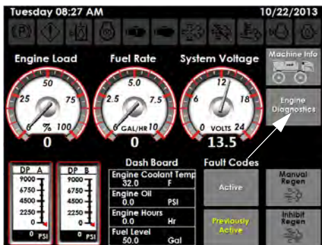
发动机诊断按钮 (位于机器诊断页面上)
