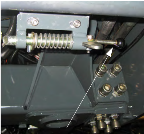
前侧加液分离杠杆 (位于机器前端下方) - 典型视图
