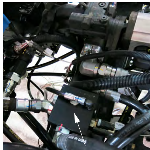
药液泵控制歧管 (位于机器中心附近) - 典型视图 * 机器上方的俯视图
