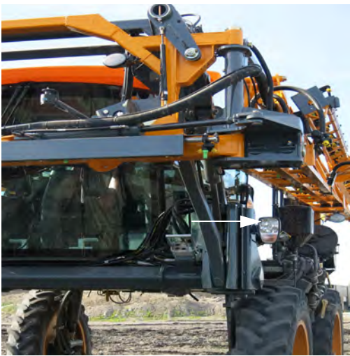
公路行驶灯 (位于驾驶室的两侧) - 典型视图
