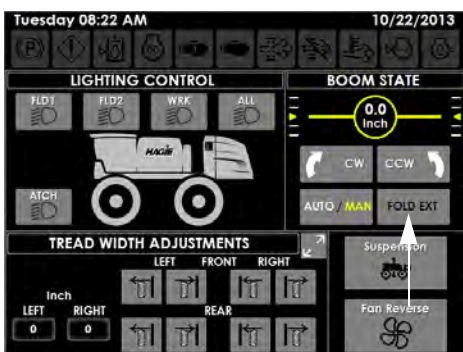
折叠伸展件 (Ext) 按钮 (位于机器显示屏辅助控制器页面上)
