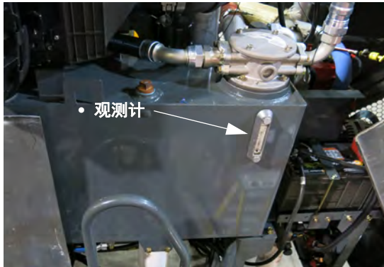
液压油箱 (位于机器左手侧 - 打开护罩后可以够着) - 典型视图
