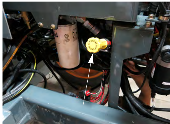
远程灌注发动机油 (位于机器左手侧 — 打开护罩后可以够着) - 典型视图
