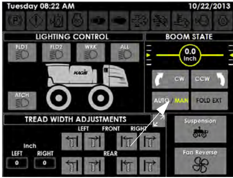
喷杆状态按钮 – 自动/手动 (位于机器显示屏辅助控制器页面上)
