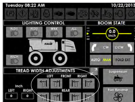
胎面调整按钮 （位于机器显示屏辅助控制器页面的底部）
