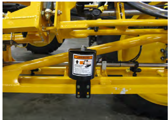
Norac 传感器泡沫垫 （位于每个 Norac 传感器上） - 典型视图
