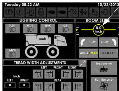
喷杆对准值 (位于辅助控制器页面的右侧)
