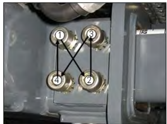
“X”顺序 - 典型视图
