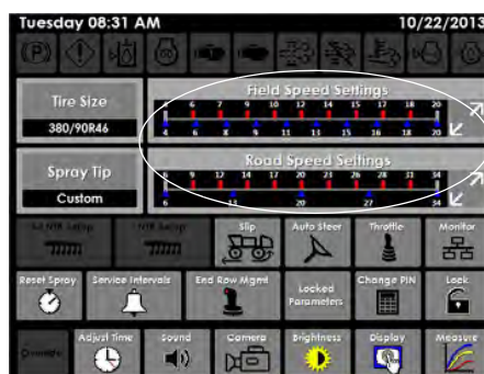
速度设置和机器调节 (位于设置页面上)
