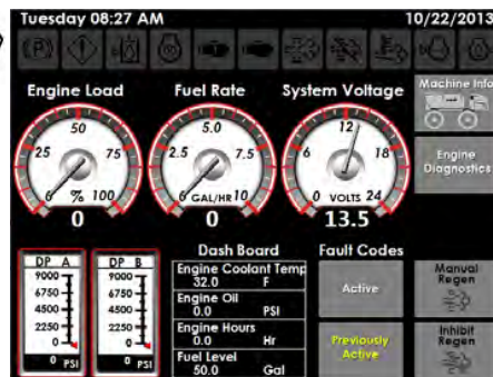
机器诊断页面
