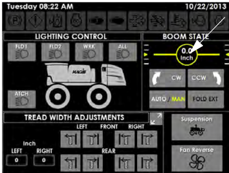
喷杆对准值 (位于辅助控制页面 右侧)
