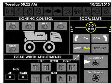
悬架按钮 (位于机器显示屏辅助控制器页面上)
