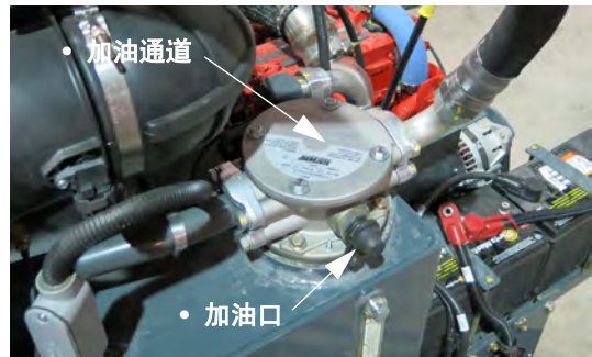
液压油灌注选项 - 典型视图
