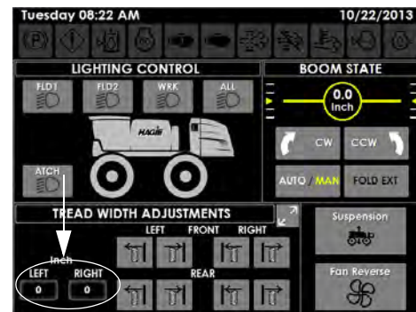
左/右胎面宽度指示器 – 后立腿 (位于机器显示屏辅助控制器页面上)
