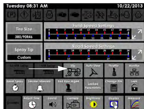
转差按钮 (位于设置页面上)
