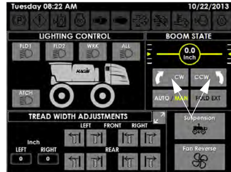
转动命令按钮 (CW/CCW) (位于机器显示屏辅助控制器页面上)
