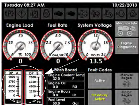
DP-A/DP-B 压力表 (位于机器诊断页面的左下侧)
