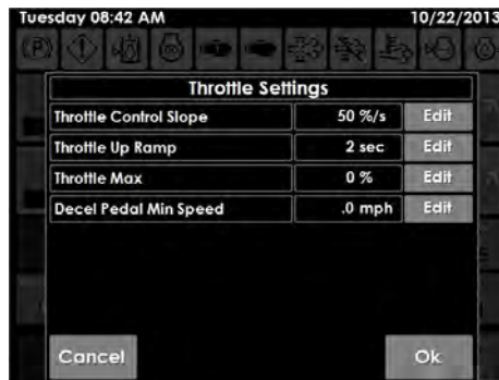
油门设置 （位于设置页面上）
