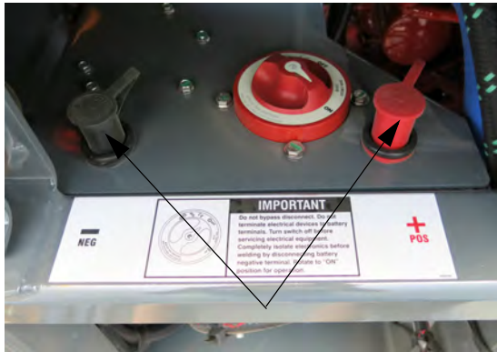
辅助电池充电接线柱 (位于后侧的主机架上) - 典型视图
