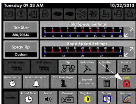
锁定按钮 (位于设置页面上)
