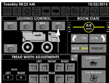
所有灯按钮 (位于辅助控制器页面上)
