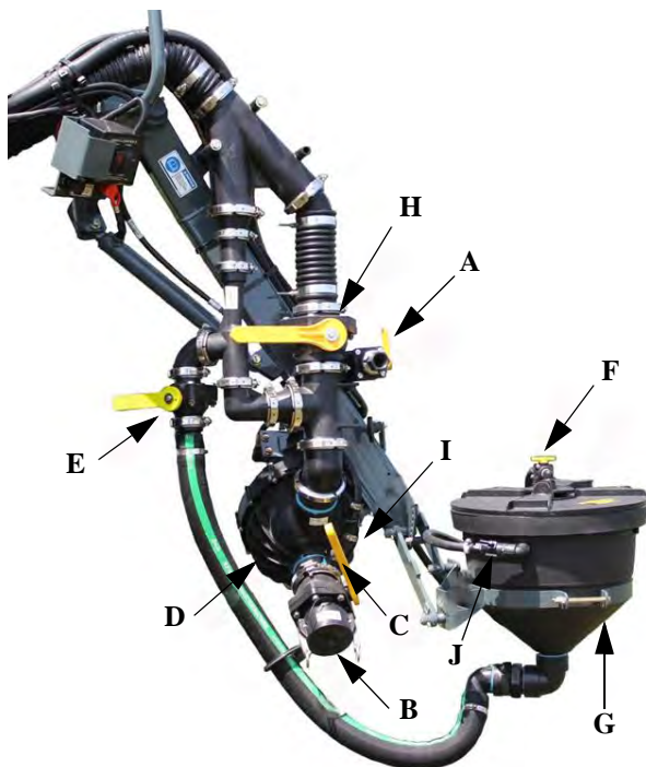
感应器总成 - 典型视图
