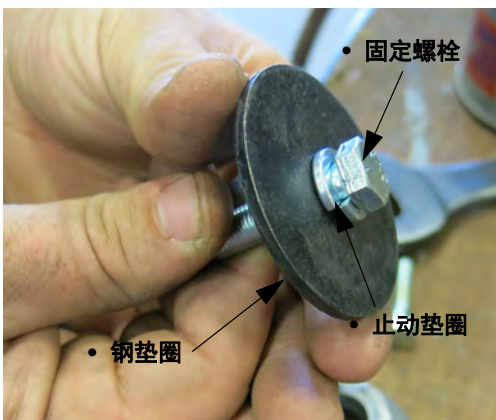
切刀螺栓/垫圈组件 - 典型视图
