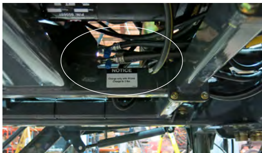
A/C 加液口 (位于主机中央之下) - 典型视图
