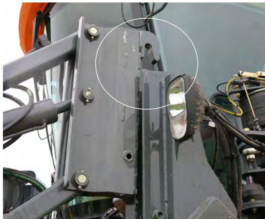
附件触及安装销 - 典型视图
