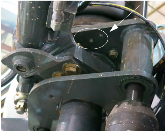
衬圈润润滑脂加油嘴 (位于每个气囊座板之下) - 典型视图
