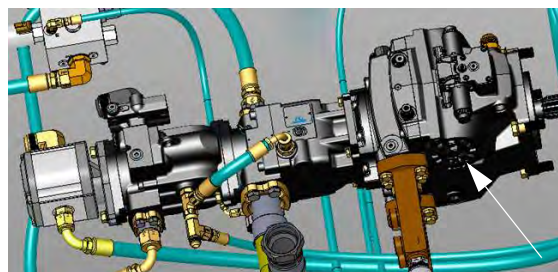
静液压泵（驱动泵） （位于发动机组的前方） * 机器上方的俯视图 - 典型视图
