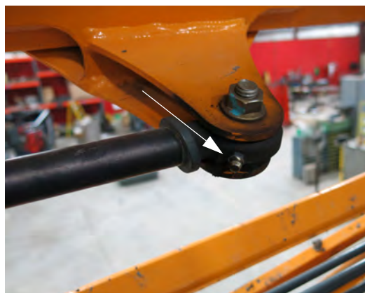
喷杆分离油缸杆端 - 典型视图
