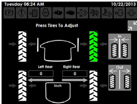
胎面调整页面
