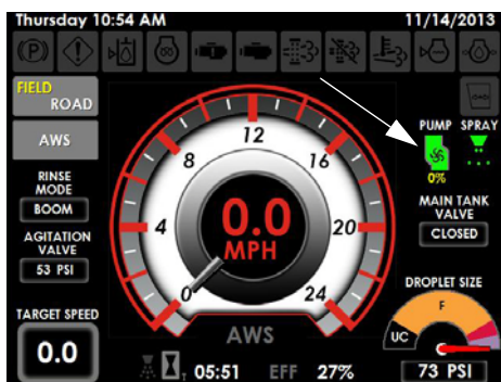
药液泵指示器 （位于机器显示屏主页 - 现场模式右侧）
