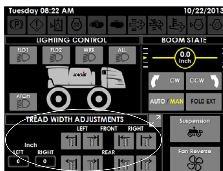
胎面宽度调节按钮/指示器 （位于辅助控制器页面上）
