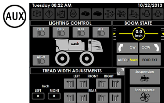
辅助控制器页面
