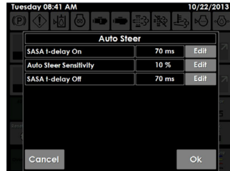
“自动转向”屏幕
