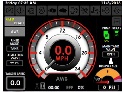
主箱阀状态指示器 (位于机器显示屏主页 - 现场模式右手侧)
