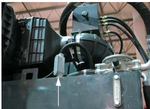
油位/温度传感器 (位于液压油箱的顶部) - 典型视图
