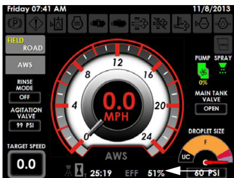
喷药效率 (EFF) (位于主页 - 现场模式上)
