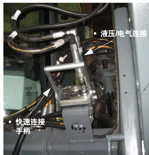
液压/电力多功能联结器总成 - “如已配置” (位于机器左前侧)
