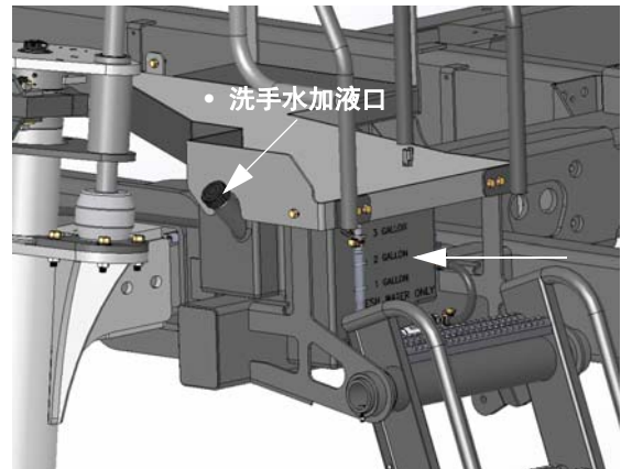
洗手水箱 (位于通道靠近梯下方) - 典型视图
