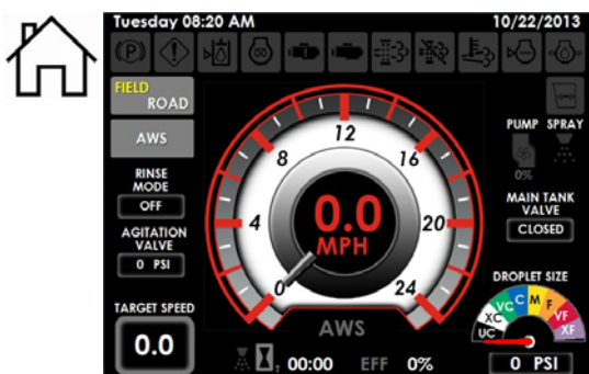
主页 (现场模式)
