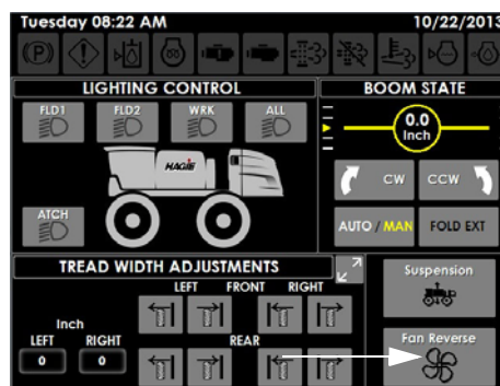
可逆转风扇按钮 （位于辅助控制器页面上）
