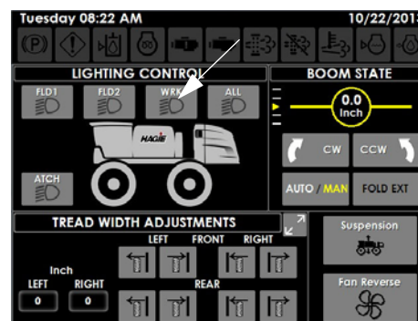
工作灯按钮 (位于辅助控制器页面上)
