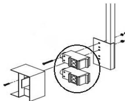
LS 光电传感器（高位/低位） - 典型视图
