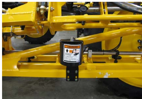
Norac 传感器 - 典型视图
