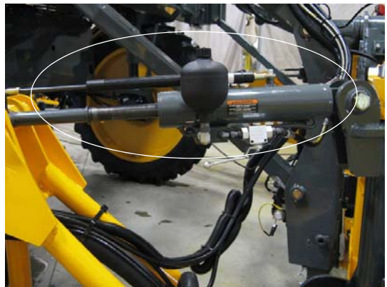
调平油缸 - 典型视图
