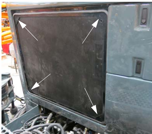
散热器护屏插销 (位于护屏每个拐角处) - 典型视图
