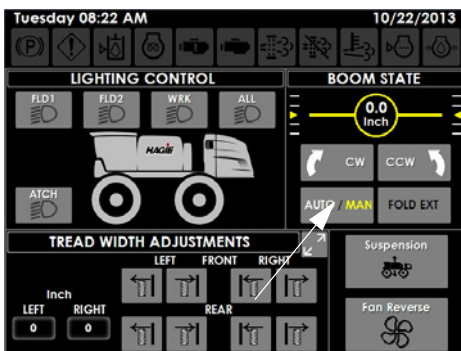
喷杆状态按钮 – 自动/手动 (位于辅助控制器页面上)
