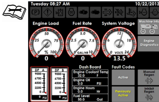
机器诊断页面
