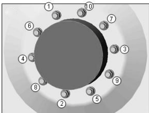
拧紧顺序
