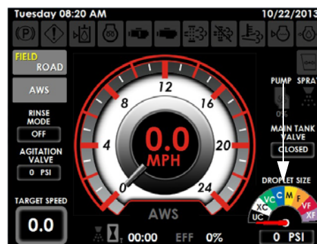
药滴尺寸指示器 (位于机器显示屏主页 - 现场模式)
