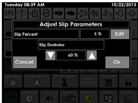
“调节转差参数”屏幕
