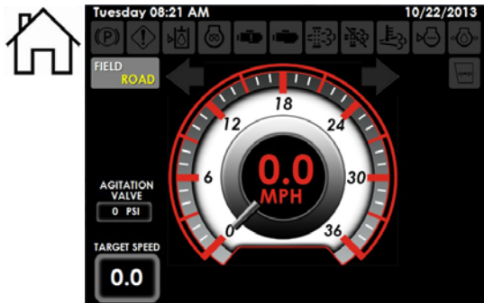
主页 (道路模式)
