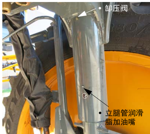
立腿管润滑脂加油嘴和卸压阀 (位于前后立腿) - 典型视图
