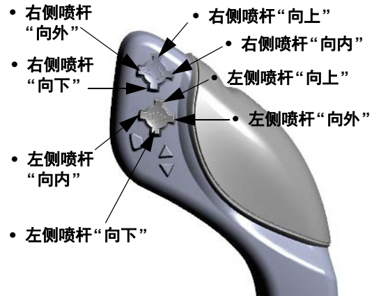
左/右喷杆开关方向 - 典型视图
