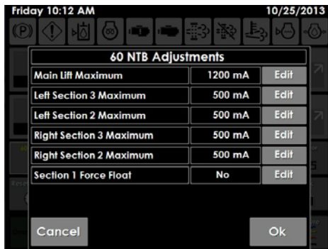
“60' NTB 调节”屏幕 - 典型视图
