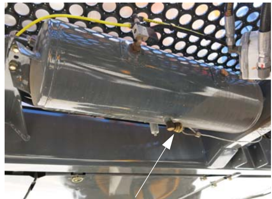
箱放气阀 (位于机器左侧通道之下) 向下拉来打开 - 典型视图
