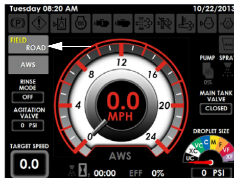
现场/道路按钮 (位于机器显示屏主页 – 道路和现场模式上)
